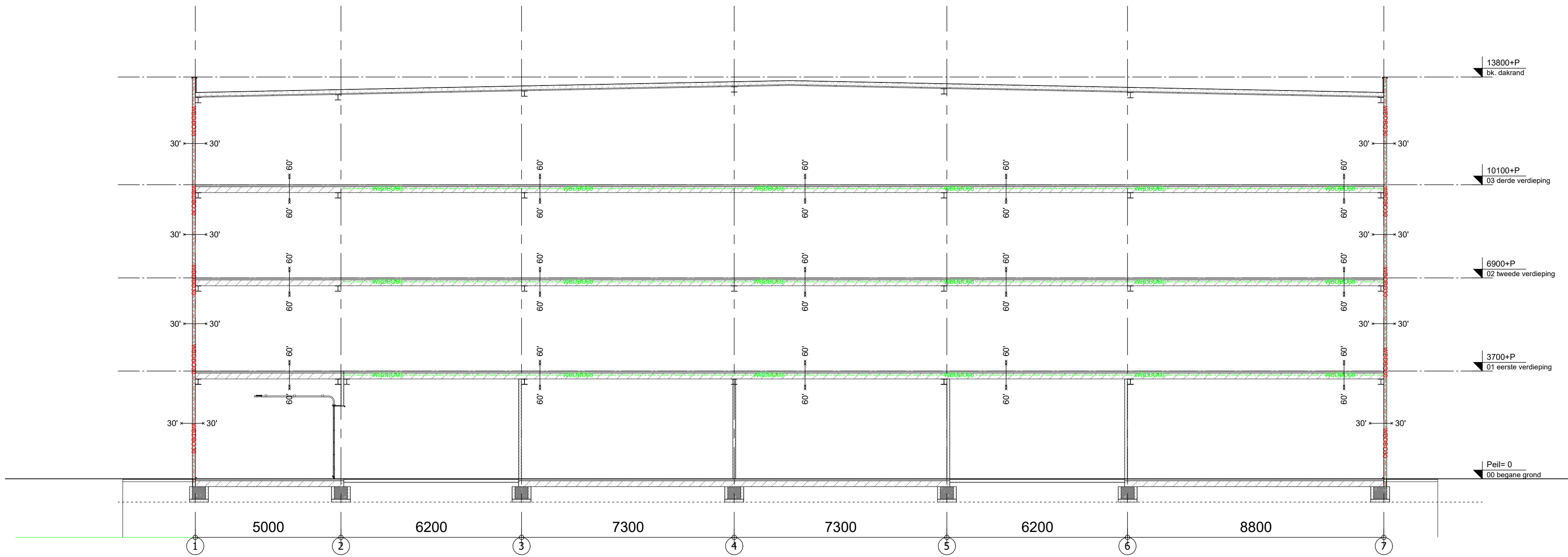
Doorsnede F-F
