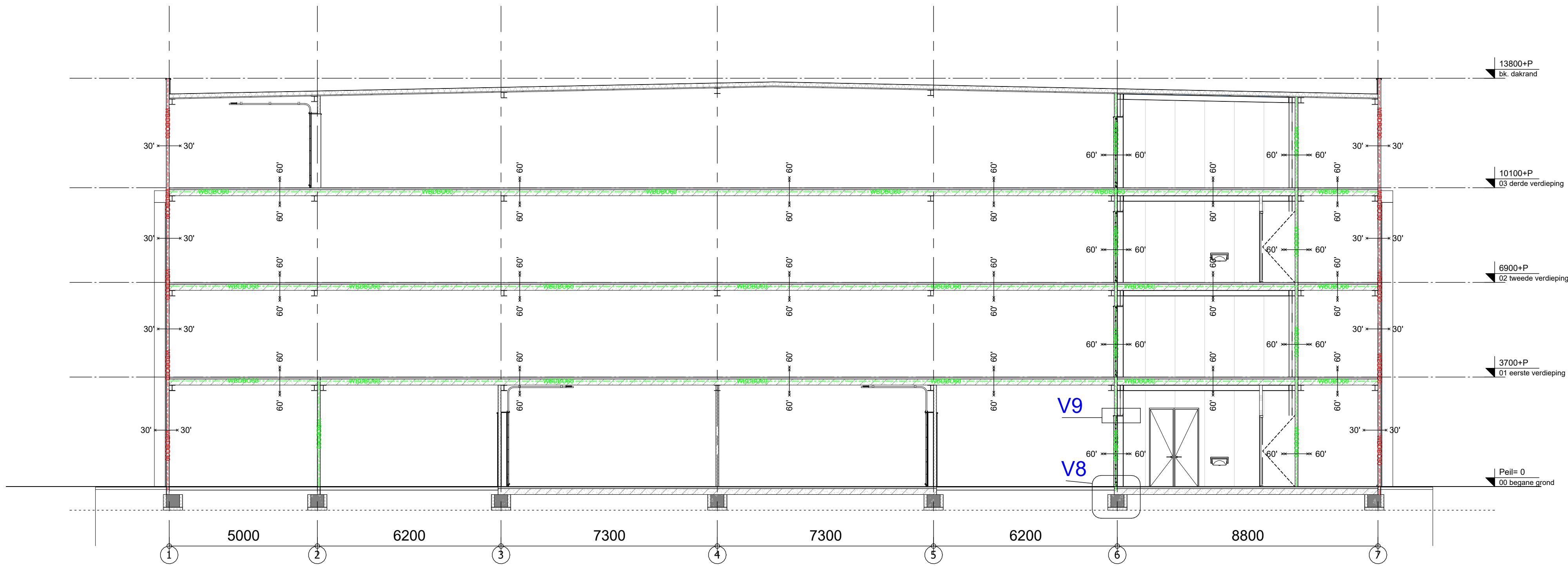
Doorsnede D-D
