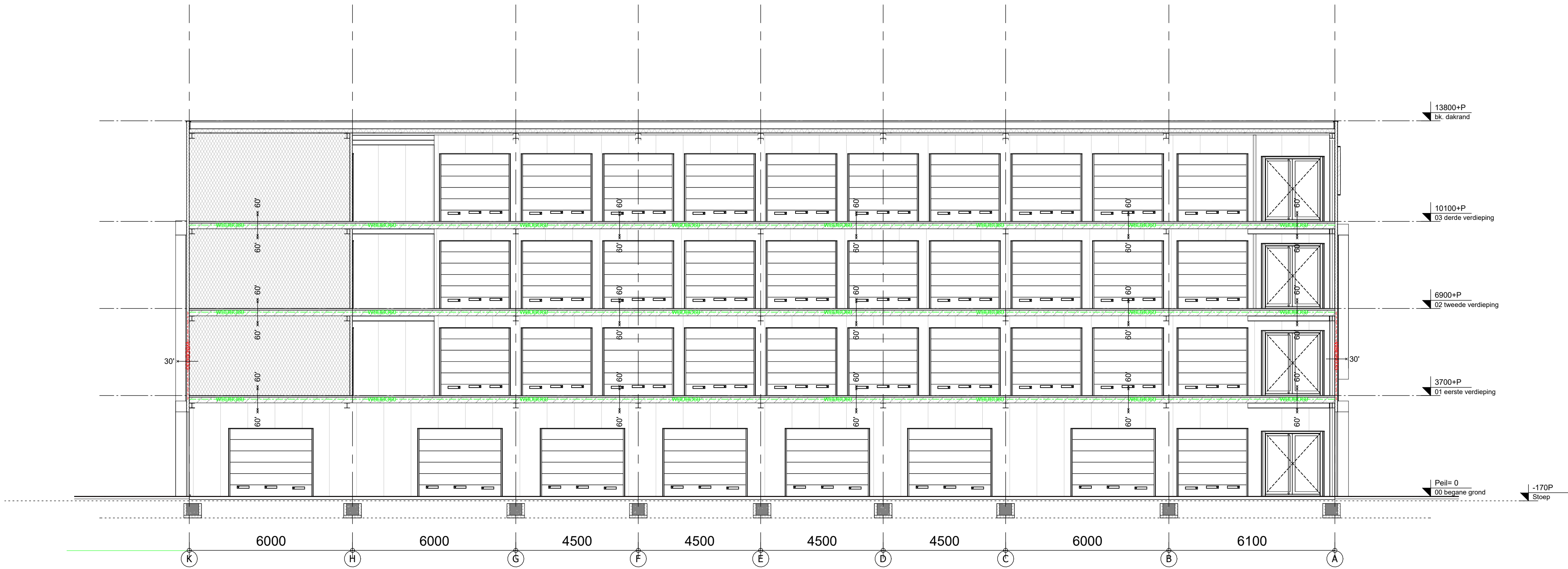
Doorsnede C-C
