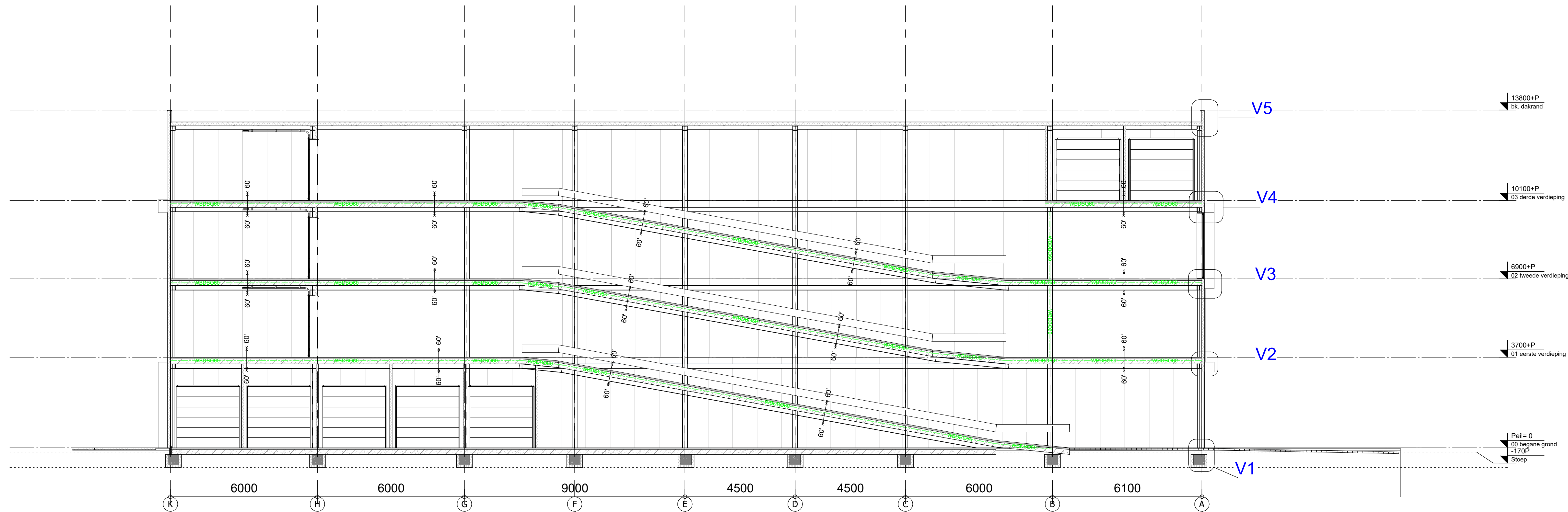
Doorsnede A-A
